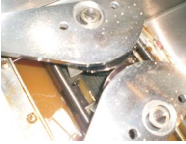
Yan tutkal sürme diskleri kitap kalınlığına göre otomatik ayarlanır
